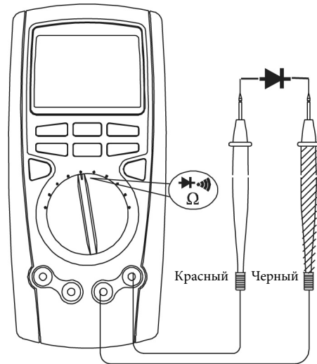
Рис. 3-5. Тест диодов
