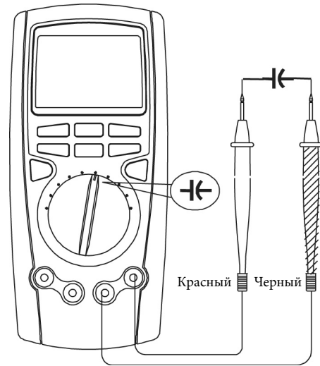
Рис. 3-6. Измерение емкости
