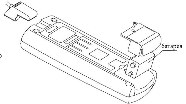
Рис. 6-2. Замена батареи
