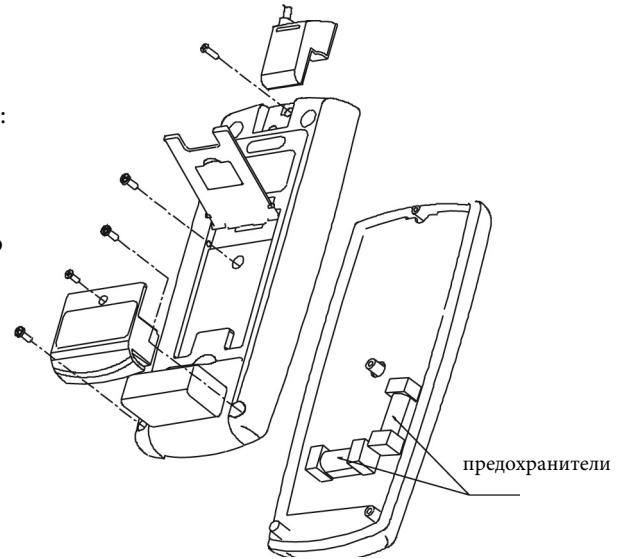
Рис. 6-1. Замена предохранителей
