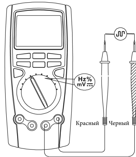
Рис. 3-7. Частота/Период измерений
