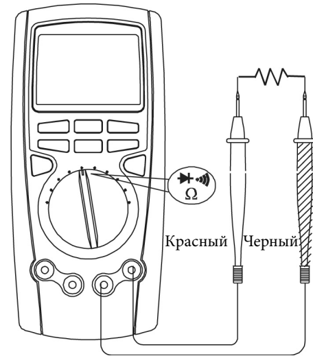
Рис. 3-3. Измерение сопротивления
