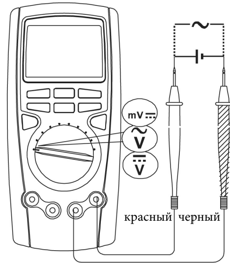
Рис. 3-1. Измерение напряжения
