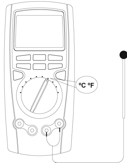
Рис. 3-8. Измерения температуры
